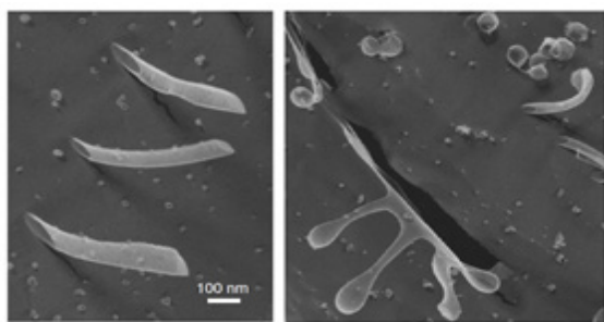
شکل ۷ نانولوله‌ها و نانوزیکول‌های تشکیل شده به وسیله پپتیدهای V6D که یک سر آب‌دوست متشکل از اسپارتیک اسید و یک دم آب‌گریز متشکل از شش اسید آمینه والین دارند [۱۵].
